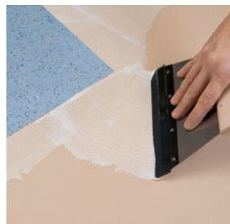
5. Cu Adezivul special LF 300 se lipesc toate tipurile de covoare, precum PVC, mochetă, linoleum.
