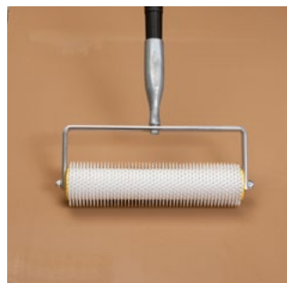
4. Se efectuează dezaerarea Șapei autonivelante rapide SL 52 , cu rola cu țepi. Această operație asigură o uscare mai rapidă a șapei autonivelante.
